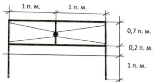
Оборудование воркаут площадки
