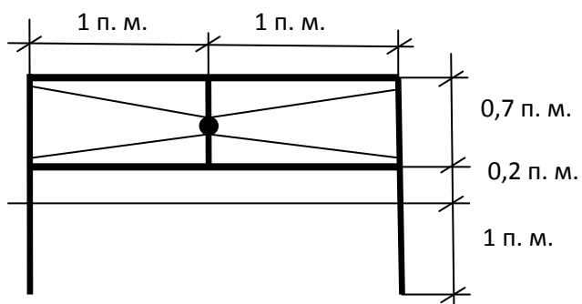
Оборудование воркаут площадки
